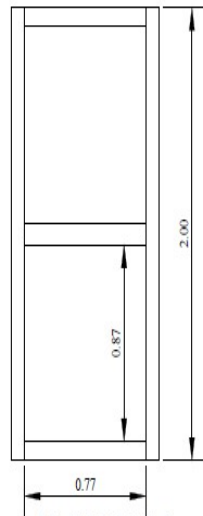
OPEN SPACE DOOR FRAME
