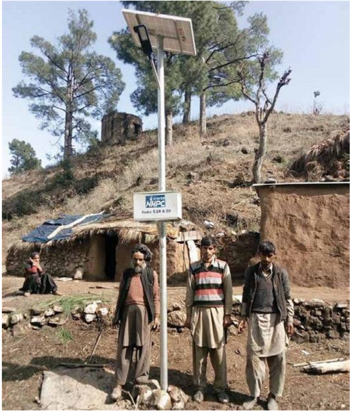
गांव आस, जिला रियासी (जम्मू-कश्मीर) के गैर-विद्युतीकृत क्षेत्रों में सलाल पावर स्टेशन द्वारा सोलर लाइट लगाना
